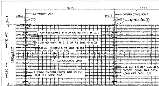
แผนแสดงการเสริมเหล็ก
